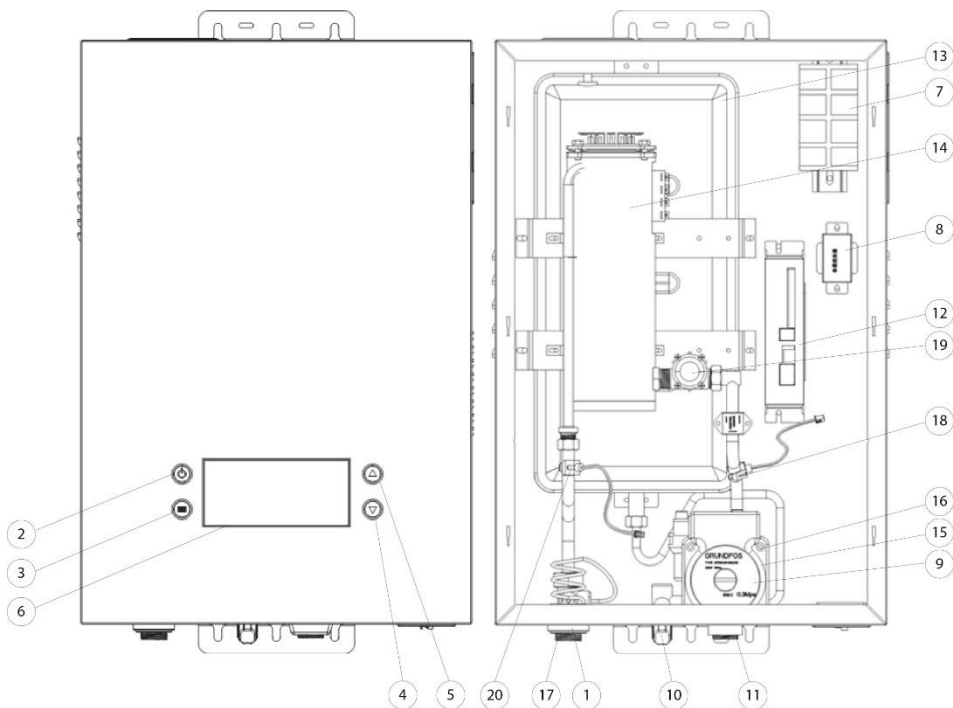
Рис. 1. Конструкция изделия
